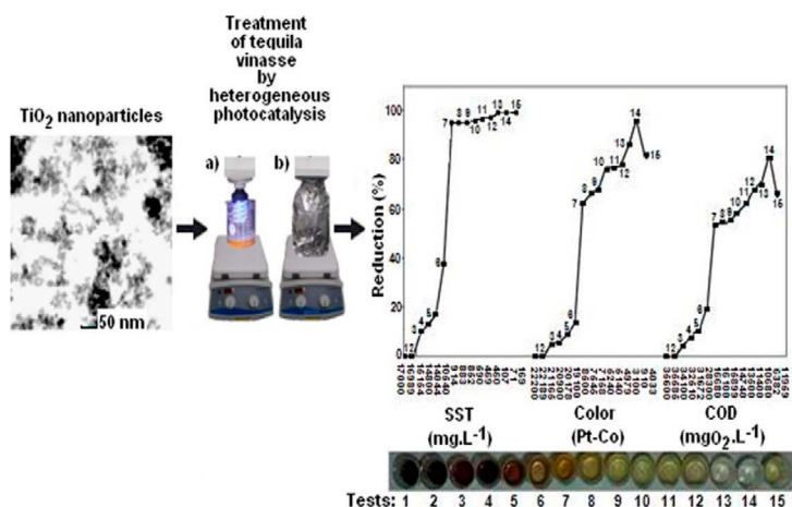
Figura 12 Fotocatálisis
